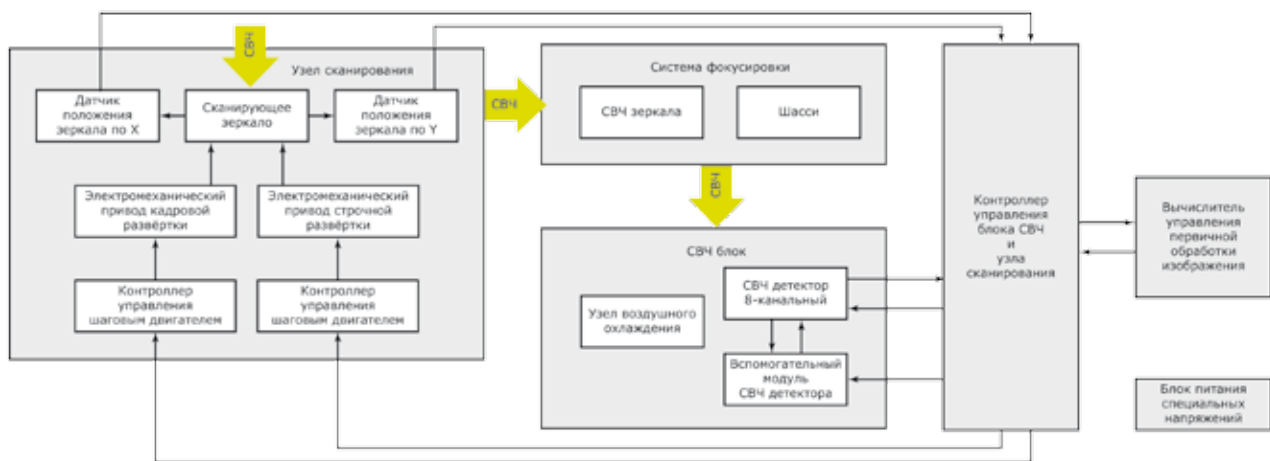
Рис. 3. Структурная схема терагерцовой камеры
