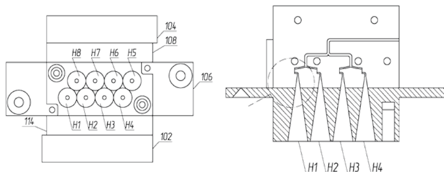
Рис. 5. Восьмиканальный СВЧ-детектор и рупорные волноводные антенны
